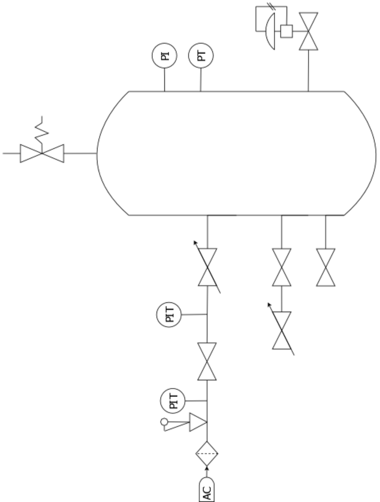
Banc de régulation de pression
